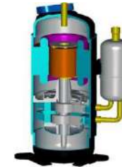
Компрессор с двойным ротором
